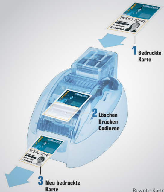
Rewrite-Kartendrucker
