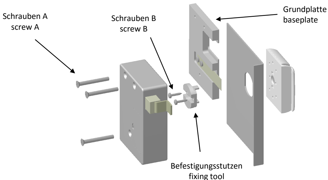
Grundplatte baseplate
